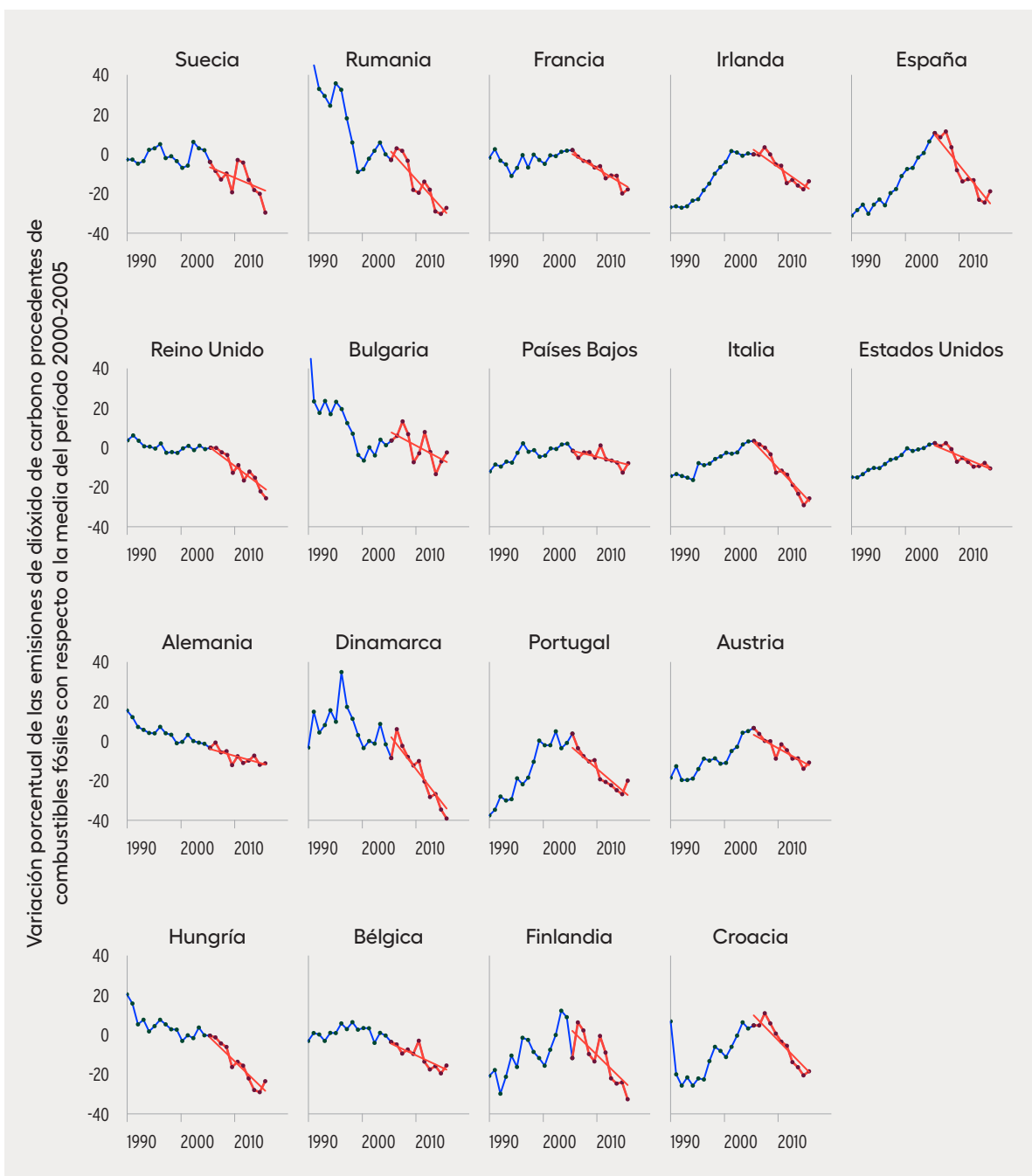
Figura 1.2 Las emisiones de dióxido de carbono procedentes de combustibles fósiles han disminuido en varios países
