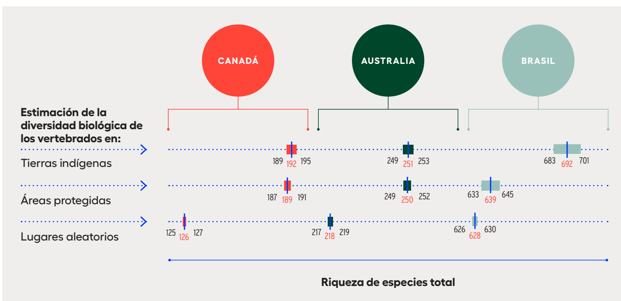
Figura 6.7 La riqueza de la biodiversidad es mayor bajo regímenes de gestión de pueblos indígenas
