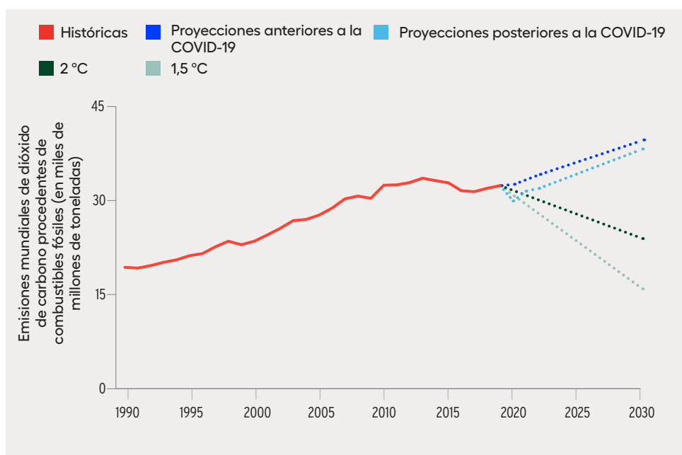
Figura S5.2.1 Es probable que las emisiones vuelvan a aumentar en 2021 a medida que las economías se recuperen y se reviertan parcialmente algunos cambios estructurales
